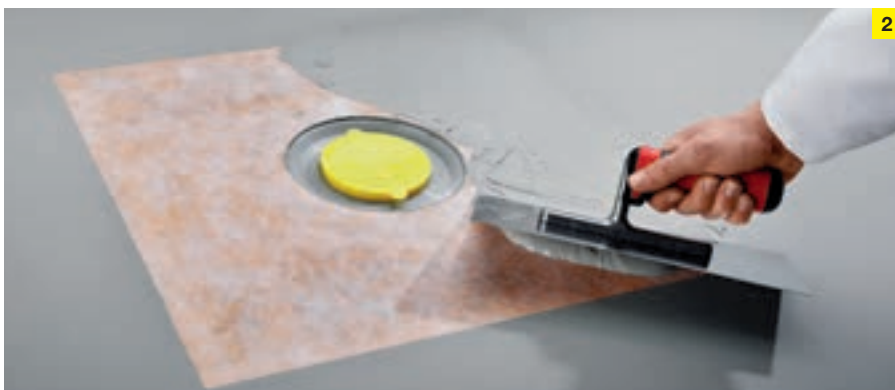
Нанасяне на 2. хидроизолационен слой с доказала се в практиката двукомпонентна комбинация от пластмаса и циментов разтвор.
